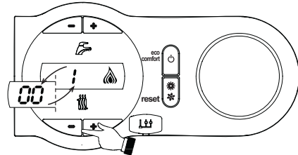
fig. 14 - Modo TEST (potencia de la calefacción = 100%)
