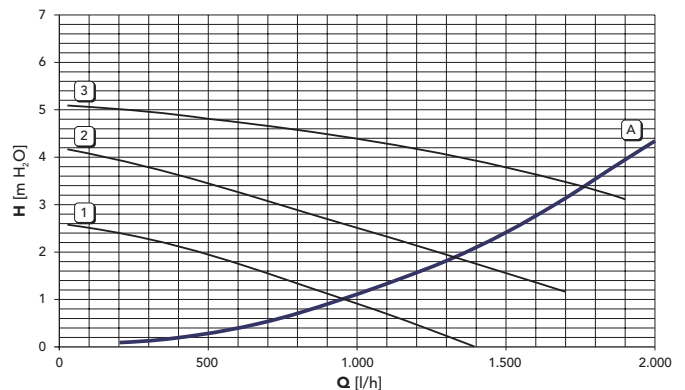
fig. 19 - Pérdidas de carga / carga hidrostática de las bombas de circulación DOMIproject F 24 D
