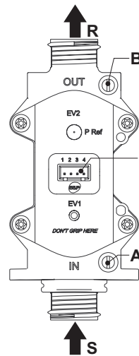
fig. 15 - Válvula del gas
