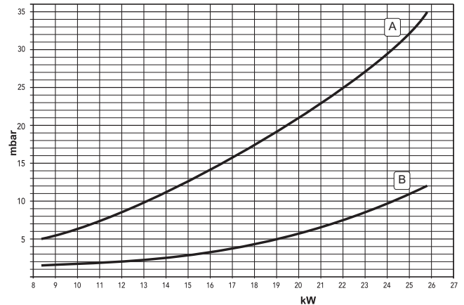
fig. 18 - Diagrama presión - potencia
